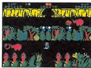
«Sabre Wulf»
